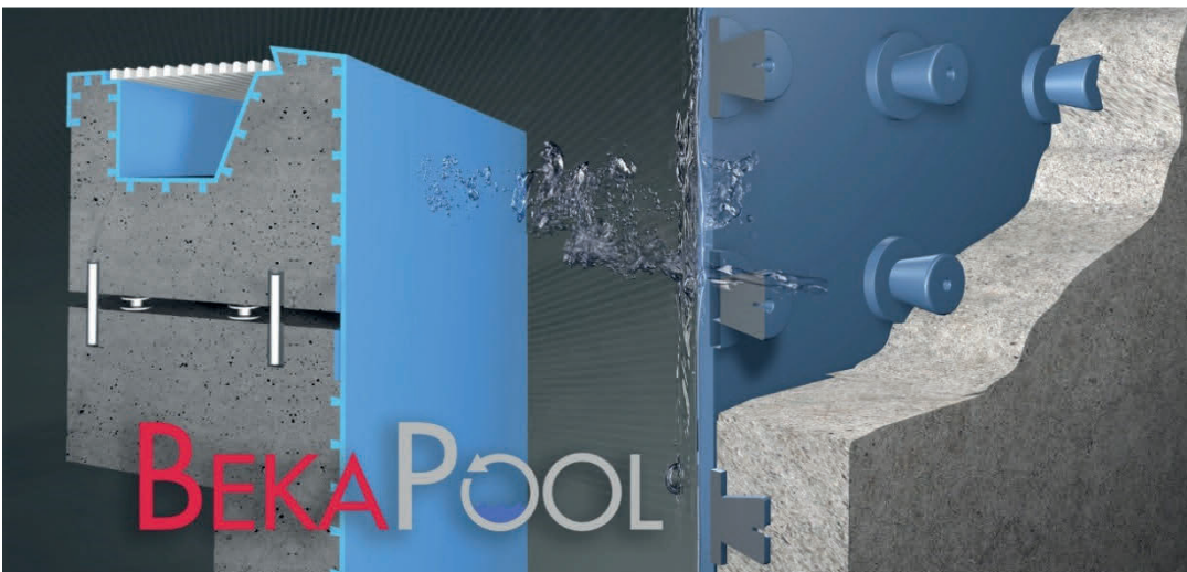
Vorgefertigter Beckenkopf mit höhenverstellbarer Überlaufrinne (links) und Systemquerschnitt der Verbundwerkstoffe. Grafik: Steuler
